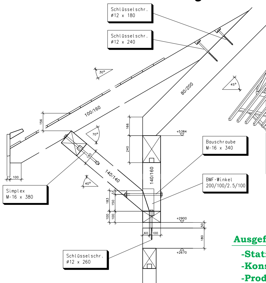
Detaile Vordach
